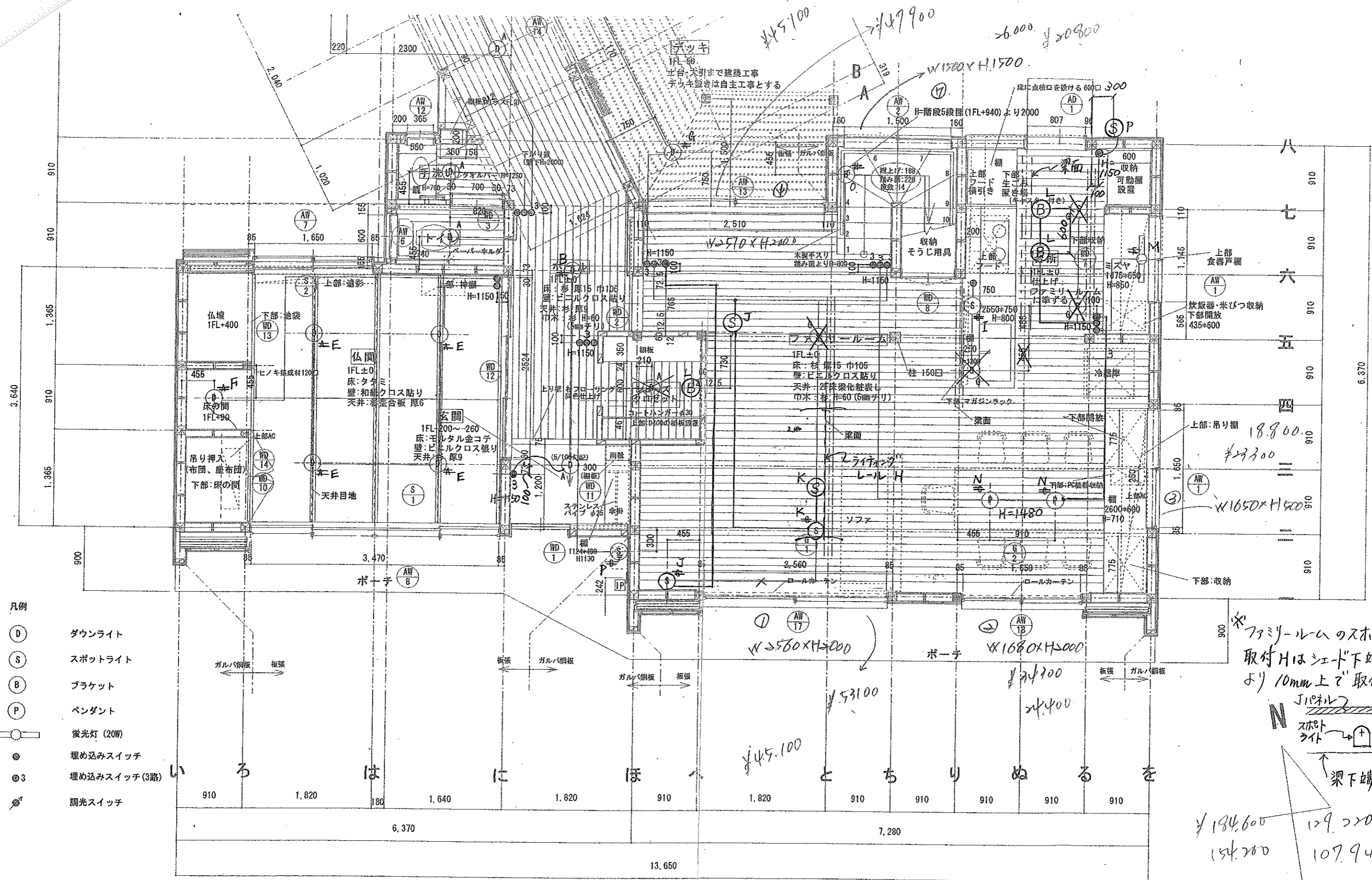
照明・スイッチプロット図 (10.12.18) 修正 (11.2.11)
